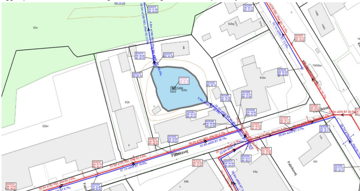
Figur 1: Tegning over regnvandssystem og søen, der anvendes som teknisk anlæg.
